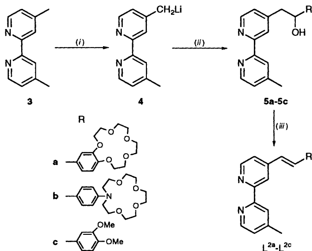
Scheme 2 (i) \text{LiNPr}^t_2 ; (ii) \text{RCHO} ; (iii) ptps
